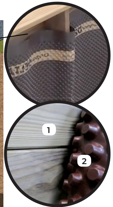
1- Armazón de composite 2- Rollo de protección y drenaje alveolar de PEHD
