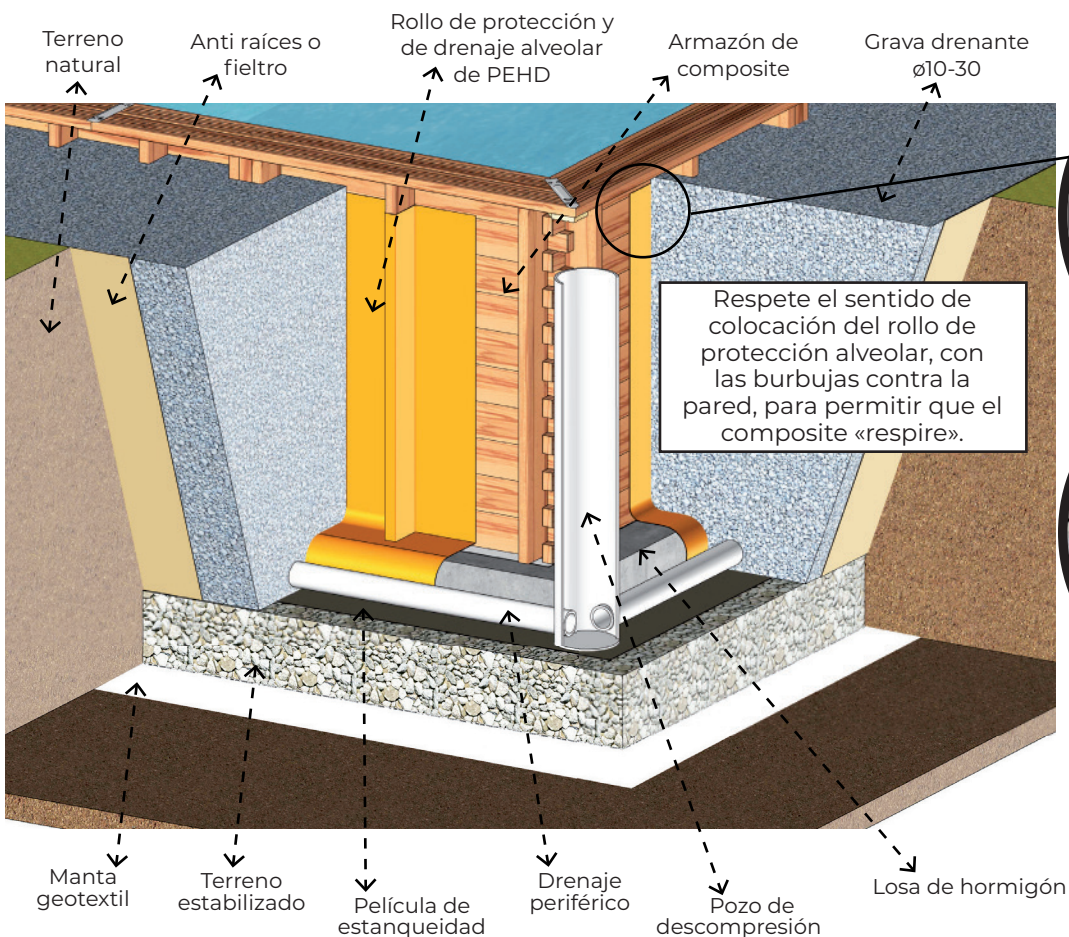
1- Armazón de composite 2- Rollo de protección y drenaje alveolar de PEHD
